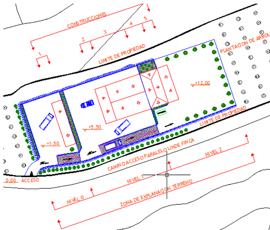
Imagen implantación edificaciones e instalaciones en la parcela con los diferentes niveles previstos
